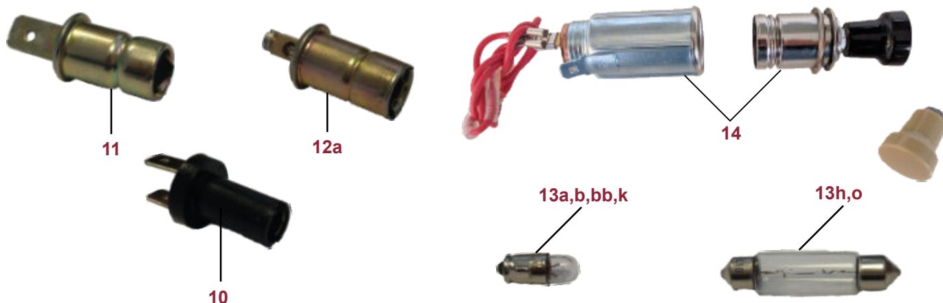
Zusammenstellung der Lampen
